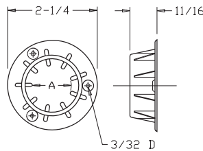
Hang Rod Flanges
